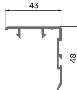
Cover profile for sash SL 39/90 Perfil de cobertura de hoja SL 39/90
