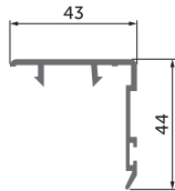
Cover profile for sash SL 39/82 Perfil de cobertura de hoja SL 39/82
